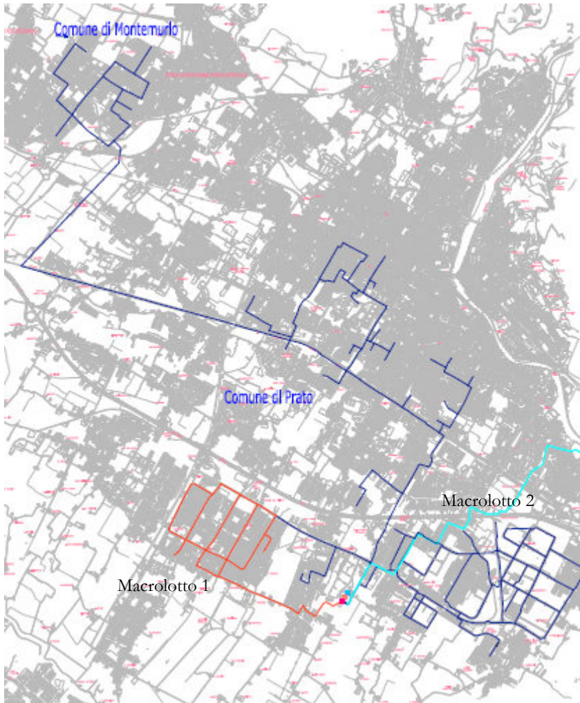
Planimetria acquedotto industriale
